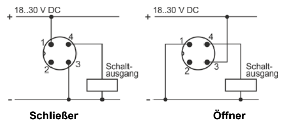
M12-Gerätestecker
