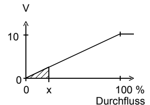
Spannungsausgang
