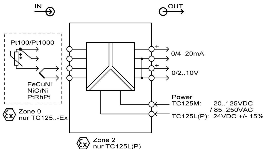
Abbildung 1 Blockschaltbild
