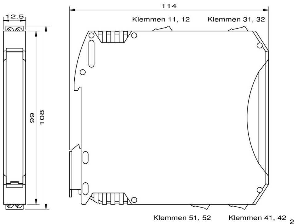
Abbildung 8 Abmessungen
