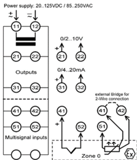
Abbildung 6 Anschlussbild
