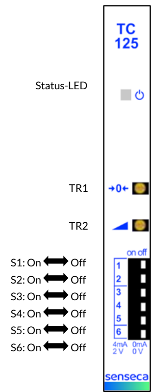
Abbildung 7 Bedienelemente
