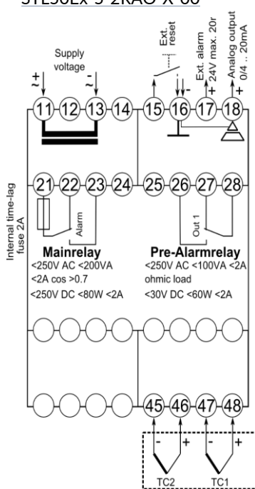
STL50Ex-5-2RAO-X-00
