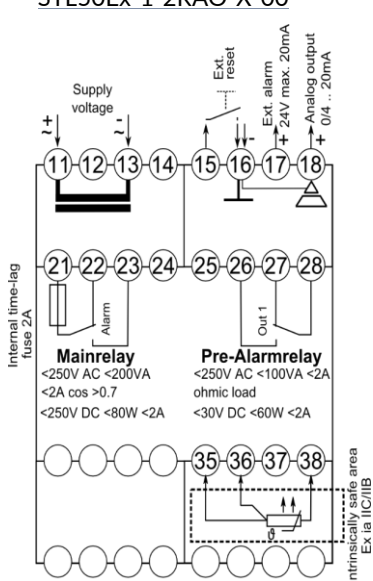
STL50Ex-1-2RAO-X-00
