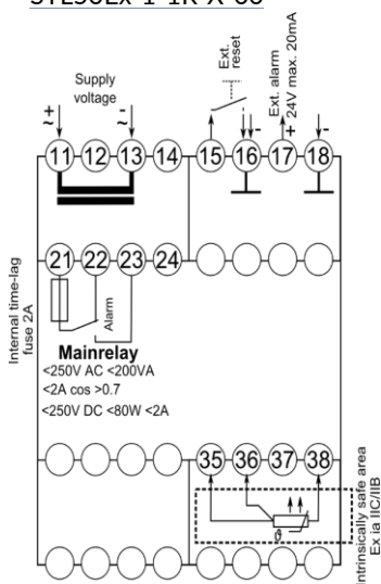
STL50Ex-1-1R-X-00
