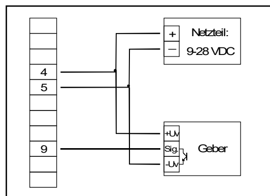
Anschluss eines Gebers (ohne eigene Versorgung) mit NPN-Ausgang
