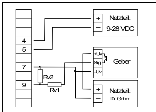
Anschluss eines Gebers (mit getr. Versorgung) PNP-Ausgang und externer Widerstandsbeschaltung
