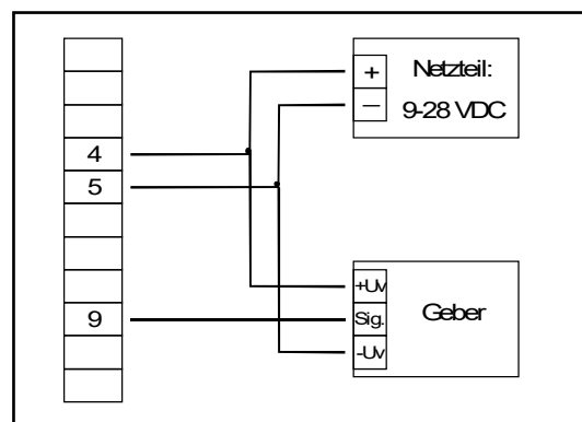
Anschluss eines Gebers (ohne eigene Versorgung) mit TTL- oder PNP-Ausgang
