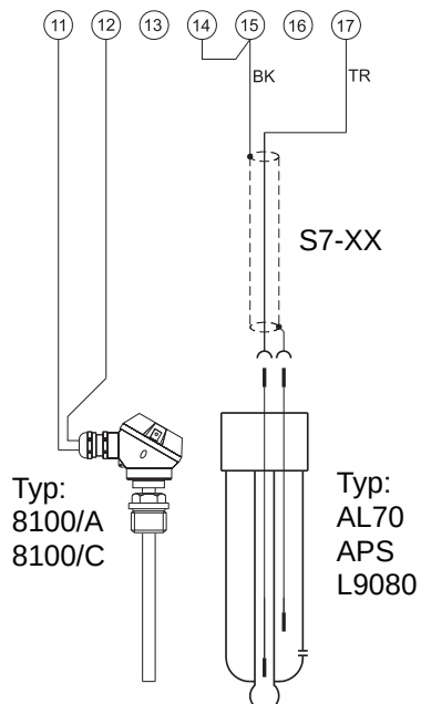
2. pH-Einstabmesskette mit ext. Temperaturfühler
