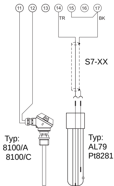
5. Redox-Einstabmesskette mit ext. Temperaturfühler
