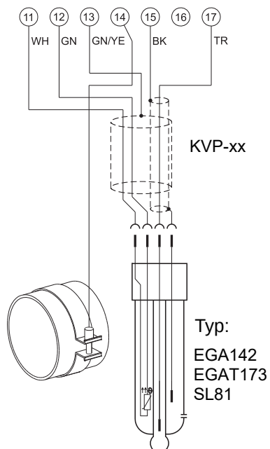
4. pH-Einstabmesskette mit integriertem Temperaturfühler und ext. Flüssigkeitserde
