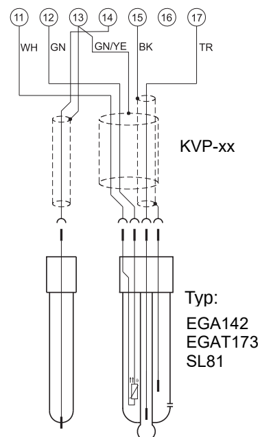
3. pH-Einstabmesskette mit Redoxelektrode
