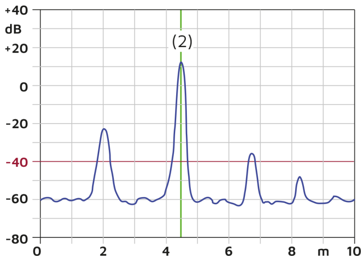
Bild 6.7: grf00047_ope_echo_curve_radar_m
