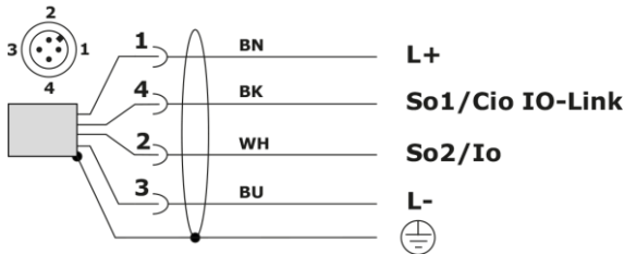
Bild 5.6: grf00031_eac_m12_4p_4w_io
