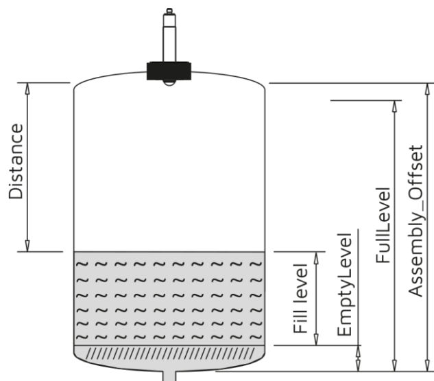
Bild 6.3: grf00041_ope_rp4ir_level
