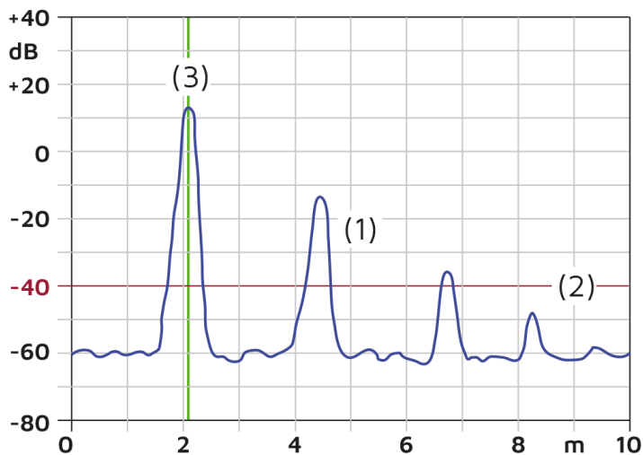
Bild 6.5: grf00045_ope_echo_curve_radar
