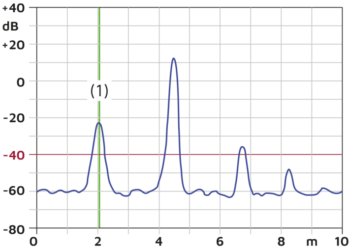
Bild 6.6: grf00046_ope_echo_curve_radar_j
