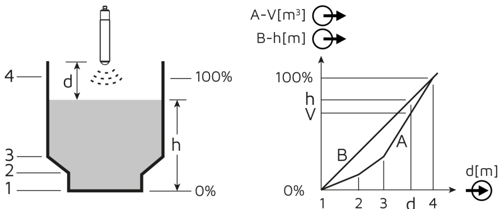
Bild 6.2: grf00044_ope_rp4ir_volume_lin
