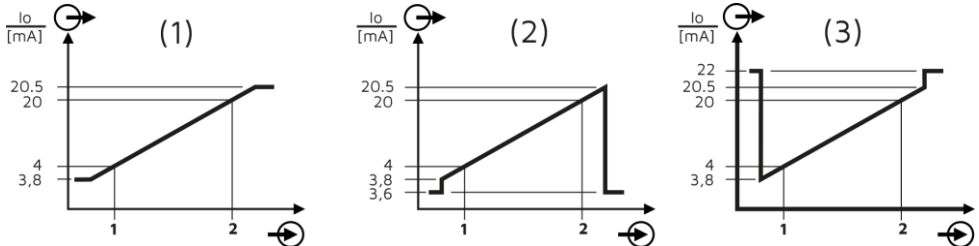
Bild 6.14: grf00054_fun_iout_4_20_h_36_22
