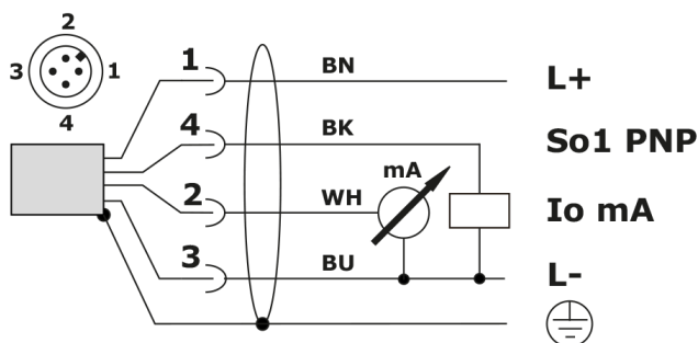
Bild 5.10: grf00036_eac_m12_4w_4w_ma_snpn
