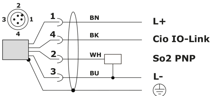
Bild 5.8: grf00034_eac_m12_4p_4w_io_snp
