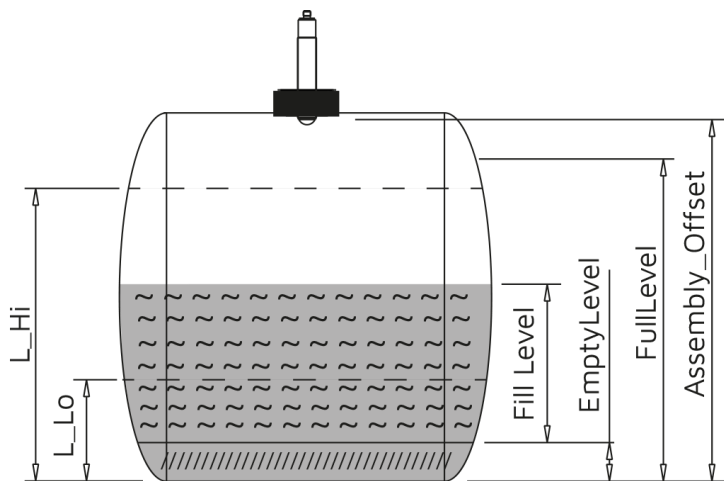
Bild 6.4: grf00042_ope_rp4ir_level_active
