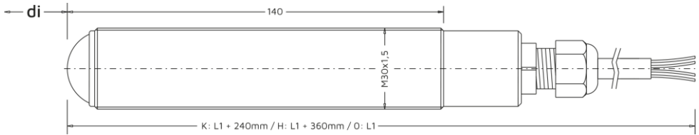
Bild 3.4: grf00023_dim_rp4sr
