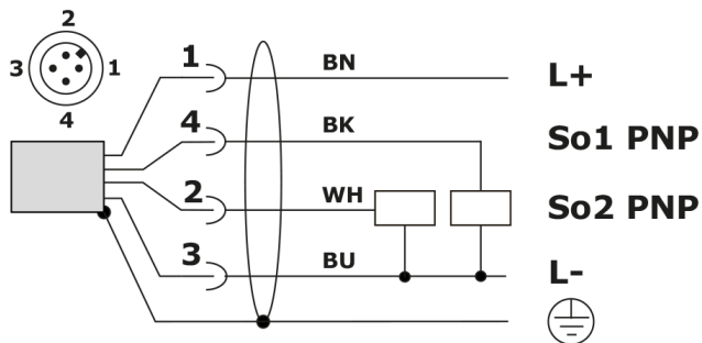
Bild 5.12: grf00038_eac_m12_4p_4w_2spnp
