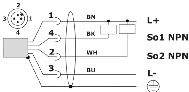
Bild 5.13: grf00039_eac_m12_4p_4w_2snpn
