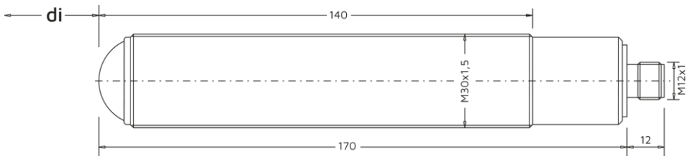
Bild 3.5: grf00024_dim_rp4ir
