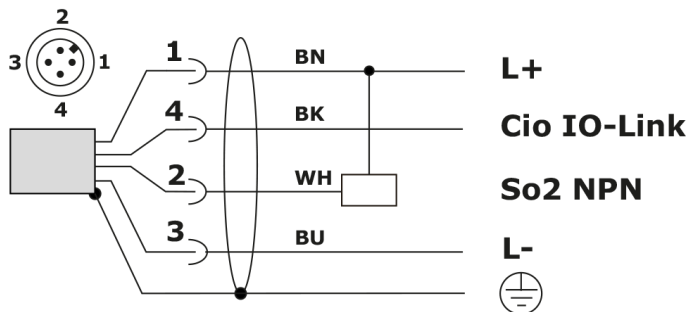
Bild 5.9: grf00035_eac_m12_4w_4w_io_snnpn
