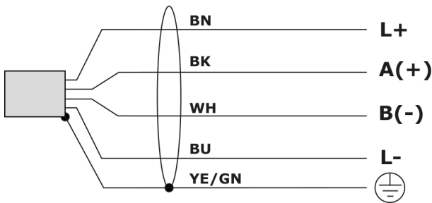
Bild 5.2: grf00028_eac_cab_4p_4w_rs485_rp4
