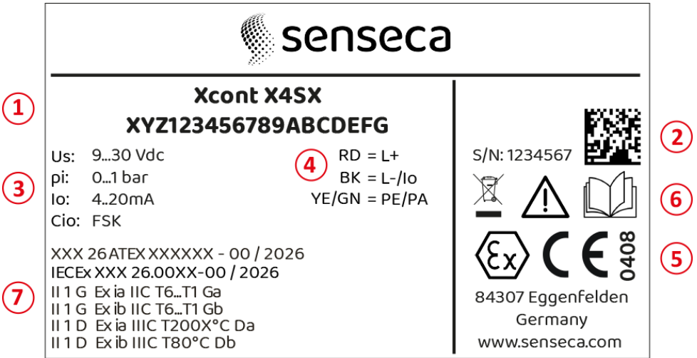
Bild 3.3: grf00002_lab001
