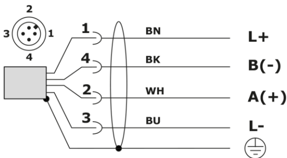
Bild 5.3: grf00029_eac_m12_4p_4w_rs485
