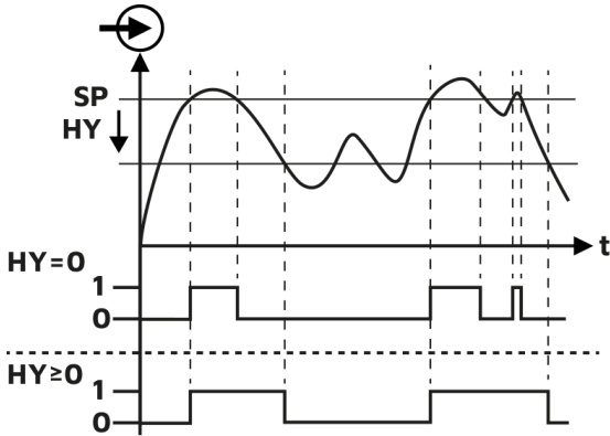
Bild 6.8: grf00048_fun_sw_sp_no
