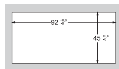
Schalttafelausschnitt
