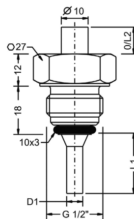
Type 4 / type 5 – Thread ISO 228-1 – G 1/2" B – front-flush gasket
