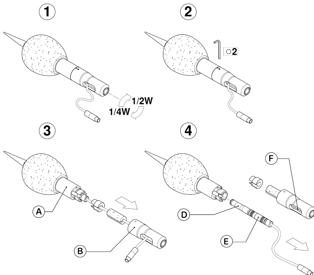
Fig. 11 - Smontaggio unità microfonica per esterni
