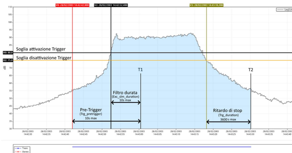
Fig. 15 - Soglia attivazione trigger
