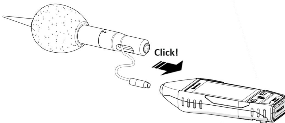
Fig. 12 - Collegamento unità microfonica per esterni
