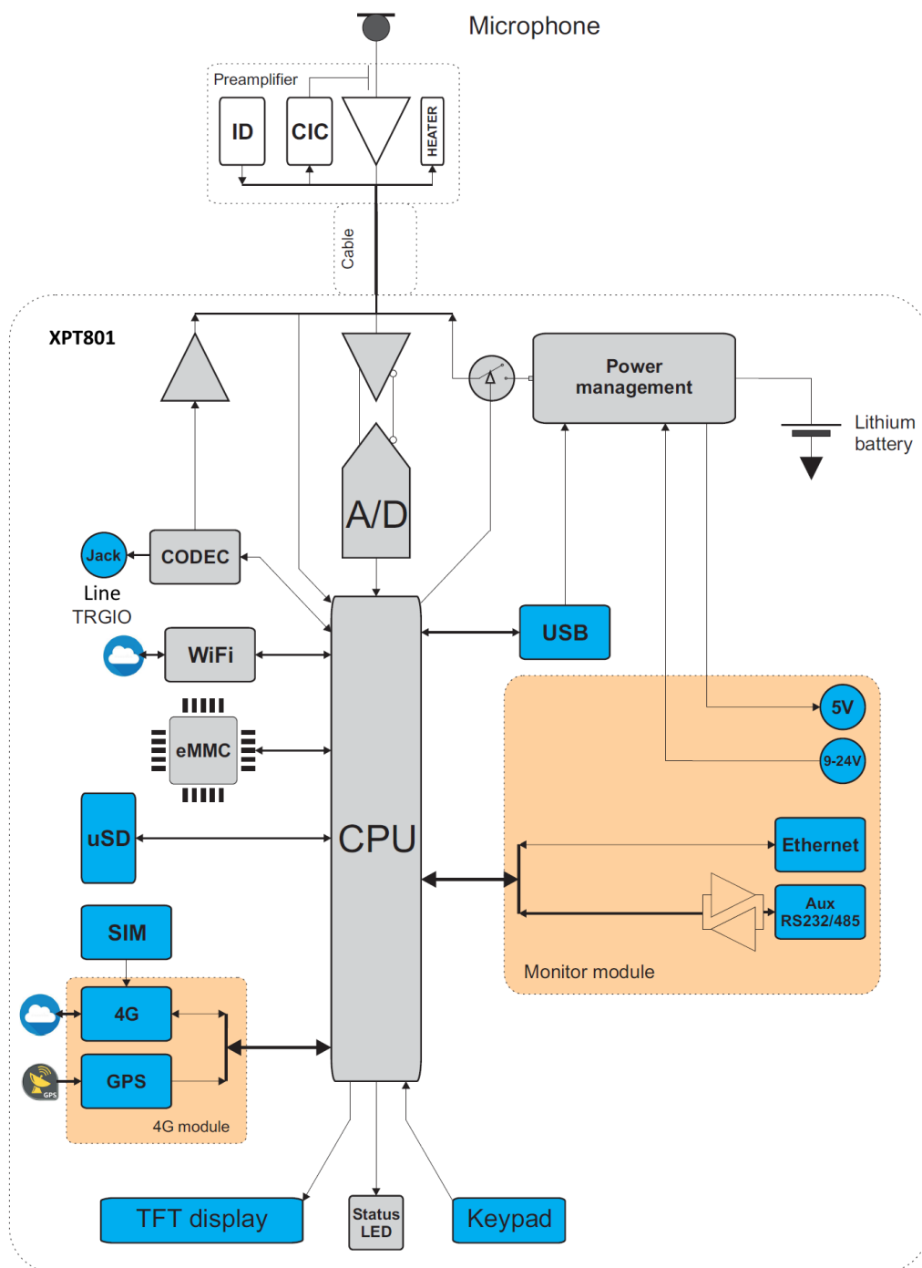
Fig. 2 - Schema a blocchi
