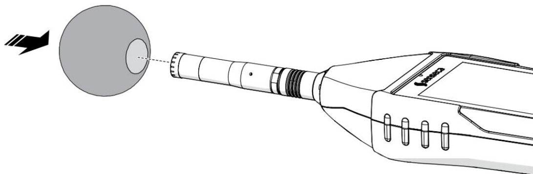
Fig. 10 - Montaggio e smontaggio schermo antivento
