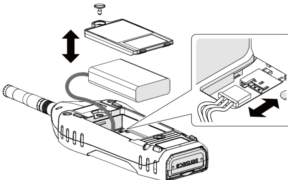
Fig. 14 - Inserimento e sostituzione della batteria
