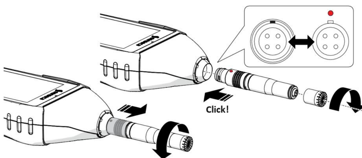
Fig. 9 - Connessione/disconnessione del microfono e del preamplificatore
