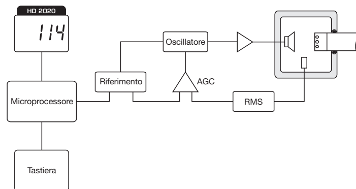
Fig. 4 Schema a blocchi della parte elettronica.
