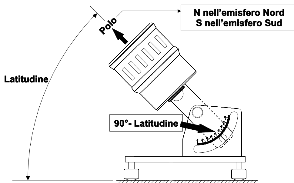
Fig. 4.6: orientazione dell'eliofanometro
