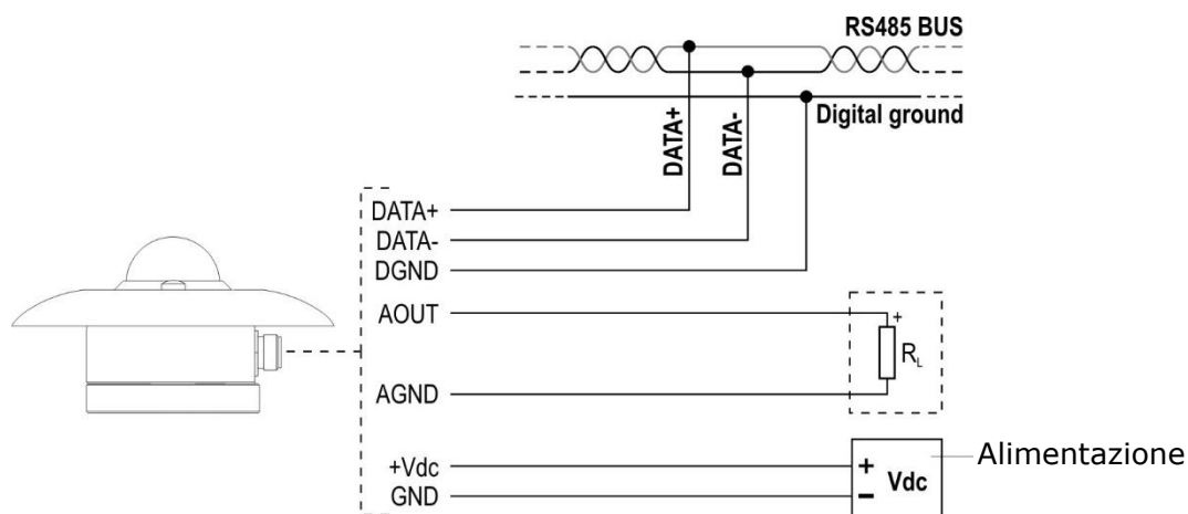
Fig. 4.4: schema di connessione LPS03Mxx
