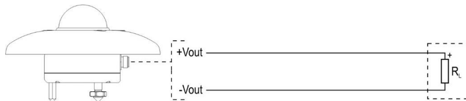
Fig. 4.6: schema di connessione LPS030P0
