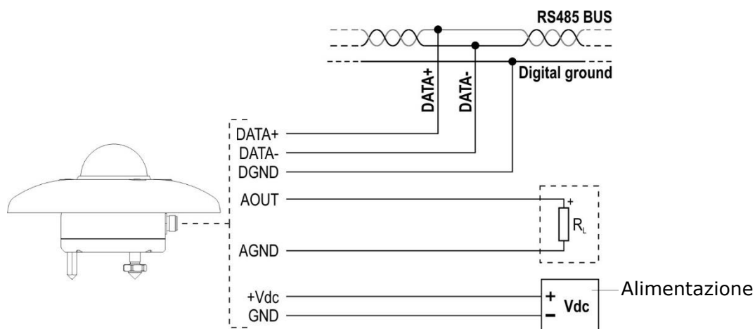
Fig. 4.4: schema di connessione LPS02Mxx
