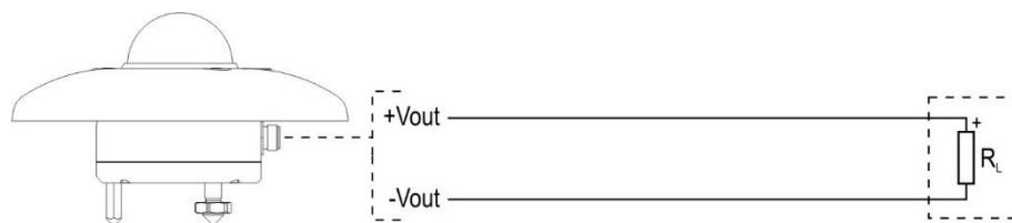
Fig. 4.6: schema di connessione LPS020P0
