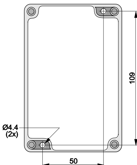
Fig. 3.1: fori di fissaggio
