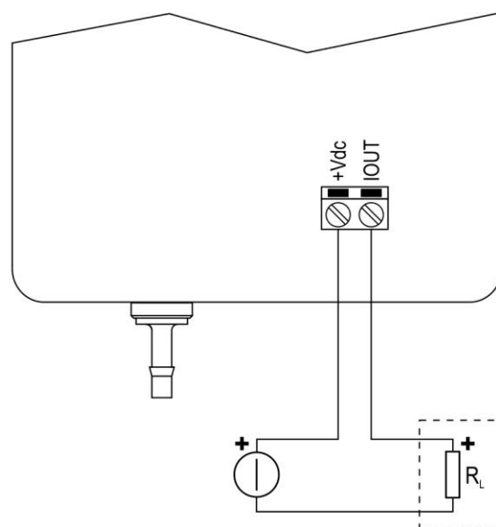
Connessione uscita in corrente
