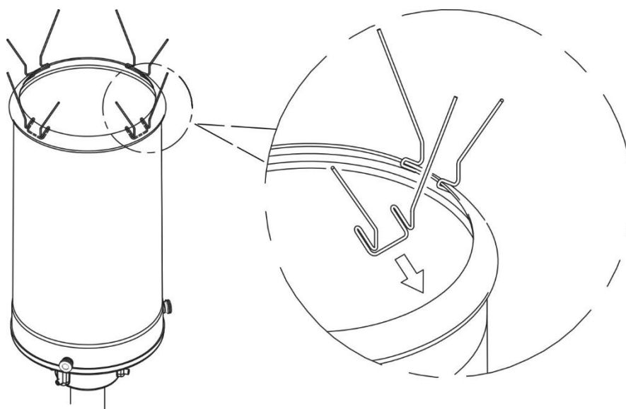
Fig. 4.4: installazione dissuasore volatili
