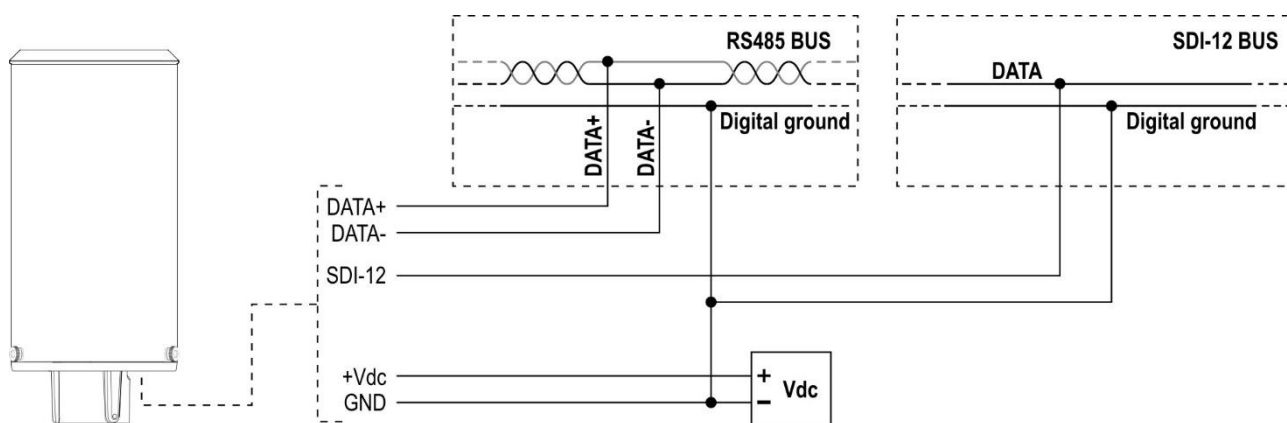
Fig. 4.7: connessione uscite digitali RS485/SDI-12
