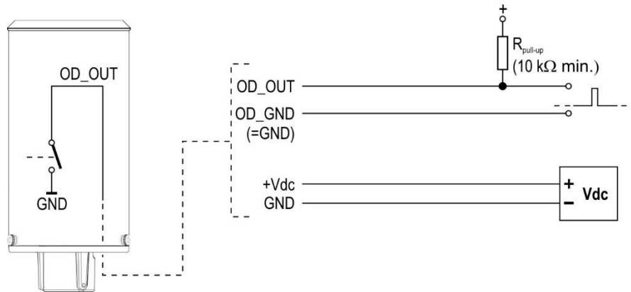
Fig. 4.10: schema di principio uscita MOSFET Open Drain
