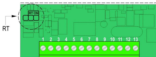
Fig. 4.8: connessione uscite digitali RS485/SDI-12
