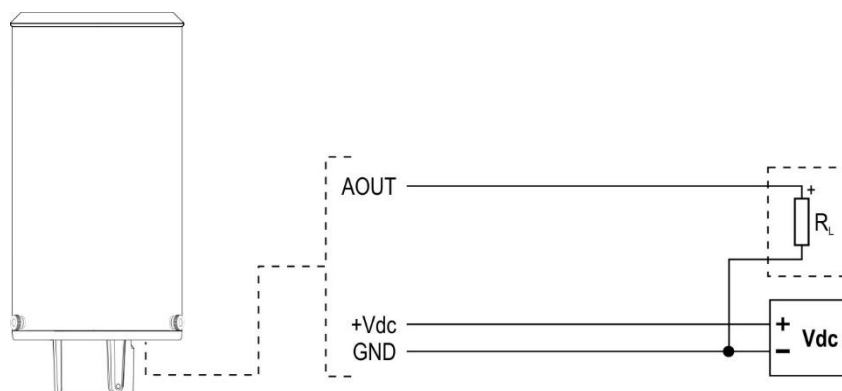
Fig. 4.9: connessione uscita analogica
