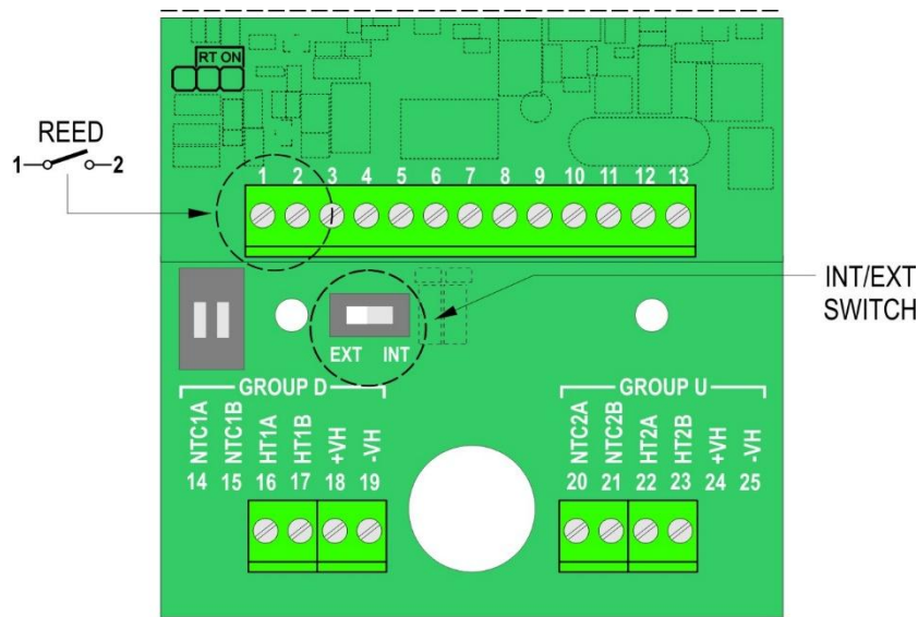
Fig. 4.5: uscita a contatto nei modelli RTD...Fx, RTD...Dx e RTD...Vx
