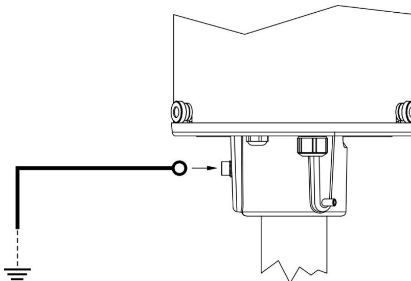
Fig. 4.13: collegamento cavo di terra
