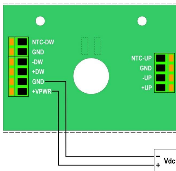
Modelli RTD...0x Morsetti a molla
