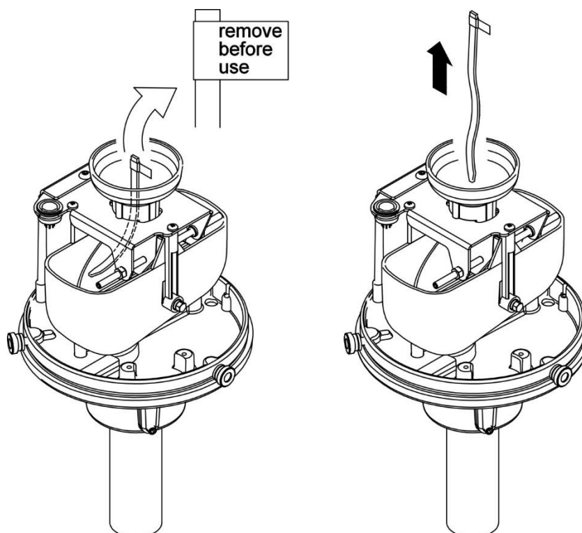
Fig. 4.14: sbloccaggio della vaschetta basculante
