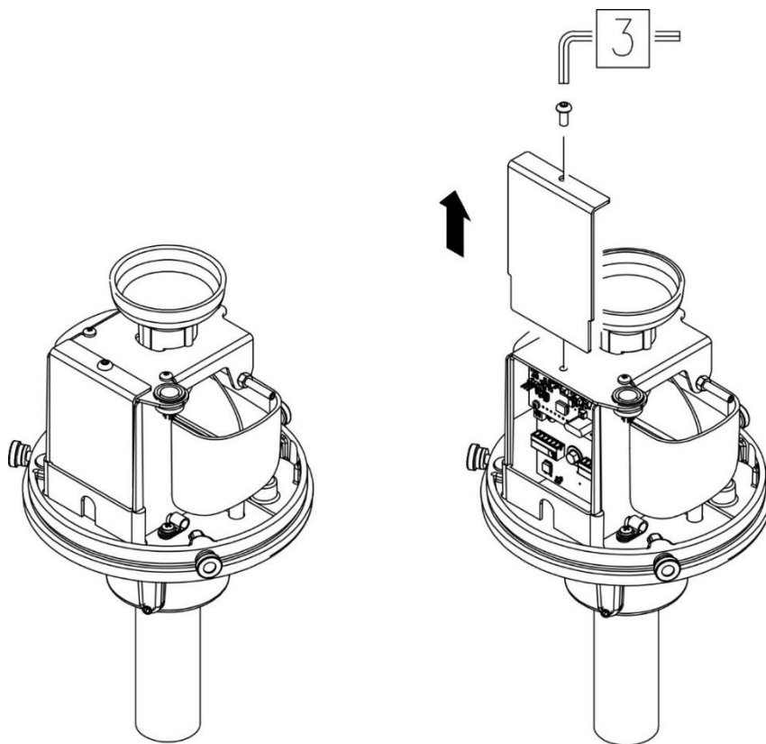
Fig. 4.11: rimozione coperchio di protezione scheda elettronica
