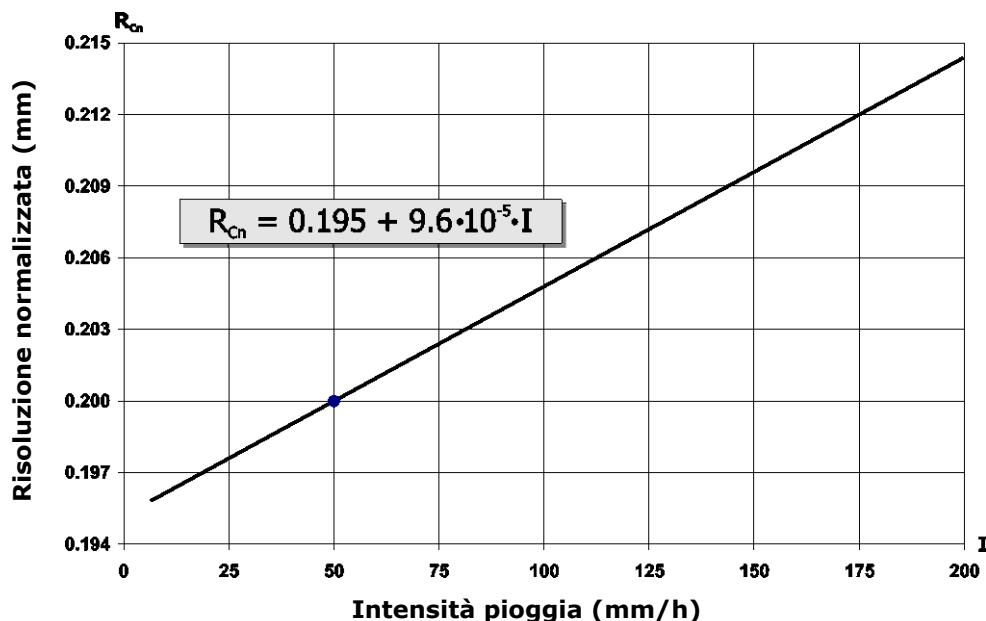
Fig. 3.1 – Risoluzione normalizzata (0,2 mm @ 50 mm/h) al variare dell'intensità della pioggia
