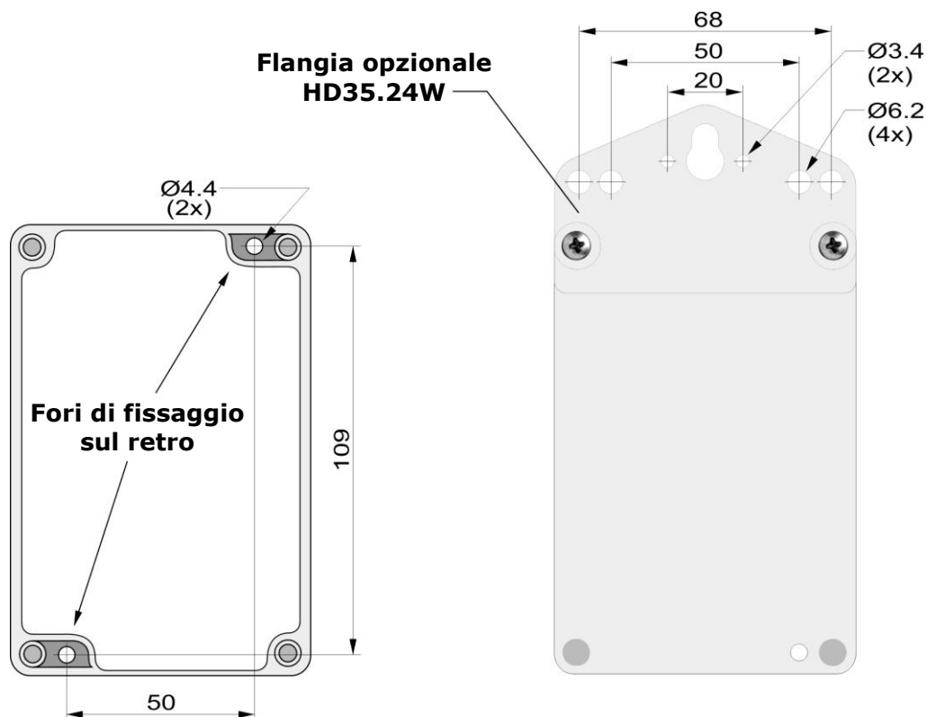
Fig. 3.3.3: modalità di installazione a parete modelli per esterni
