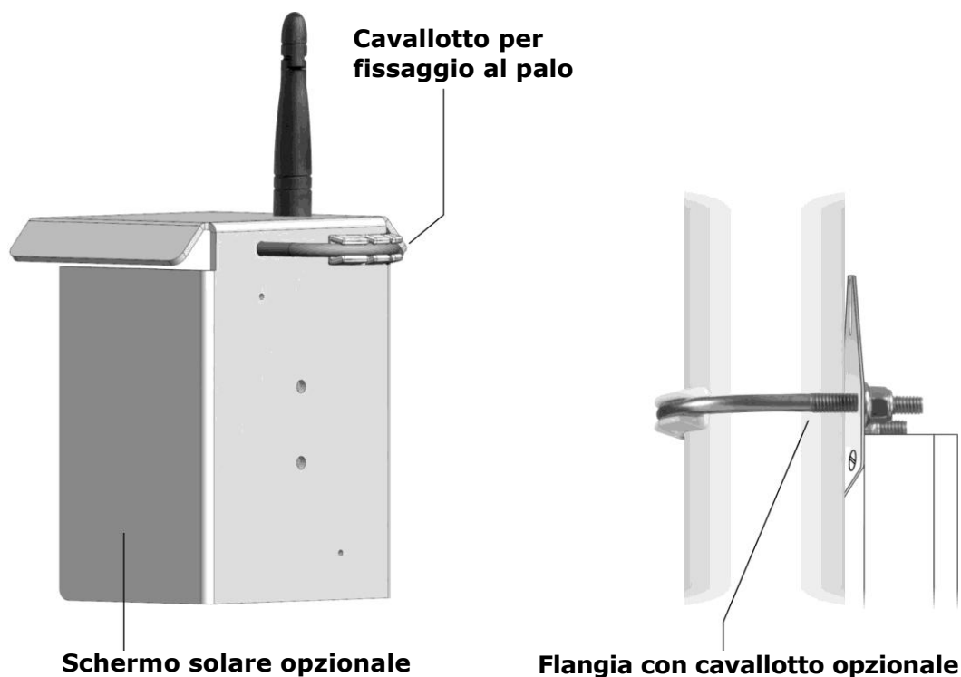
Fig. 3.3.2: modalità di installazione su palo modelli per esterni
