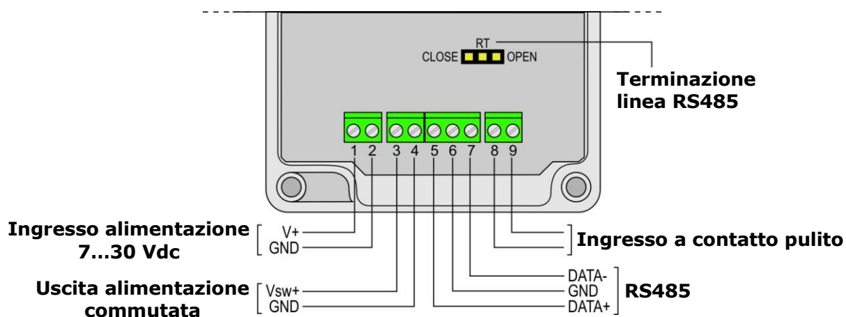
Fig. 3.7.1: connessioni LR35LW-MB
