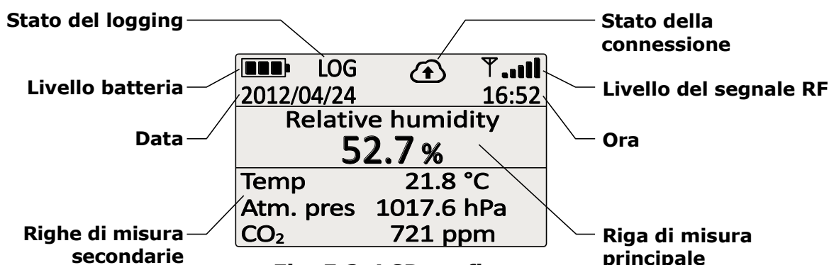
Fig. 5.2: LCD grafico
