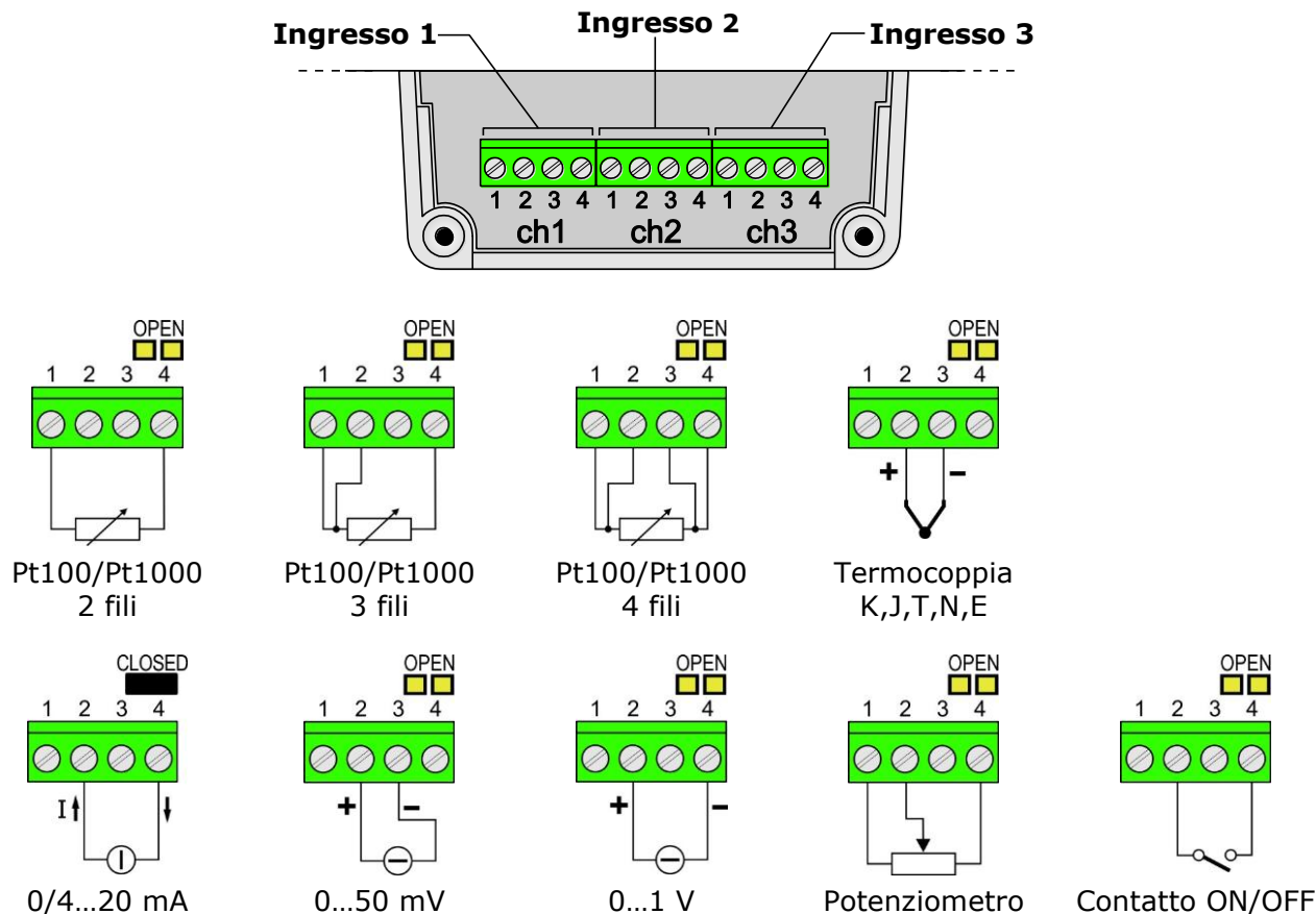
Fig. 3.5.1: collegamento dei sensori in LR35[G]H
