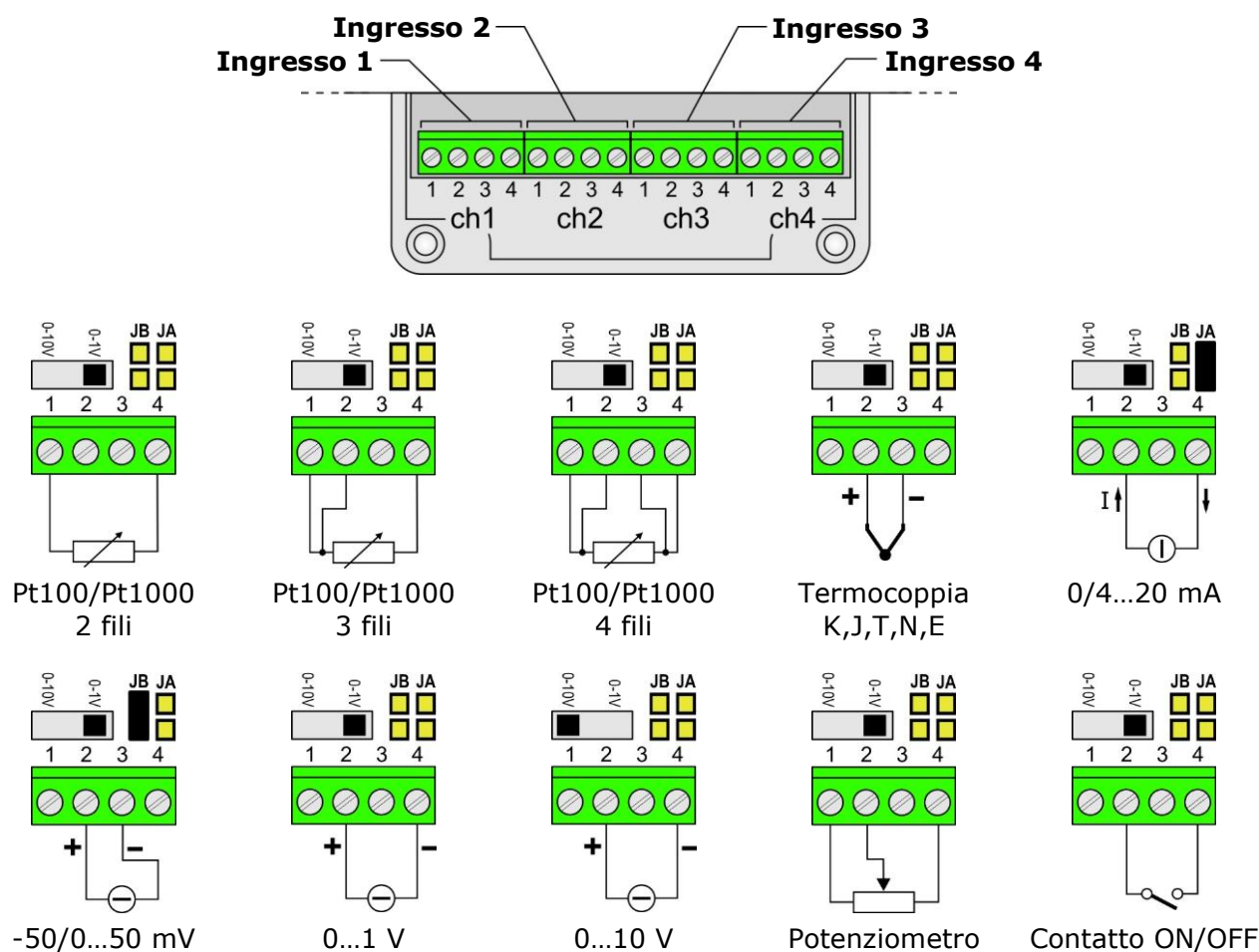
Fig. 3.6.1: collegamento dei sensori in LR35LWH
