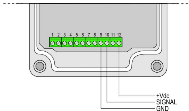
Fig. 3.8.1: collegamento sensore di livello
