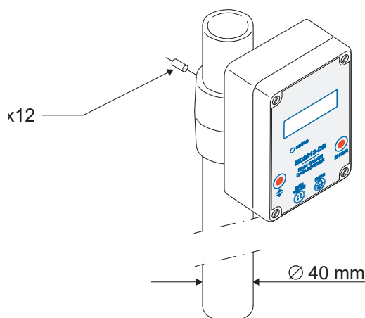
Fig.1: Installazione con manicotto
