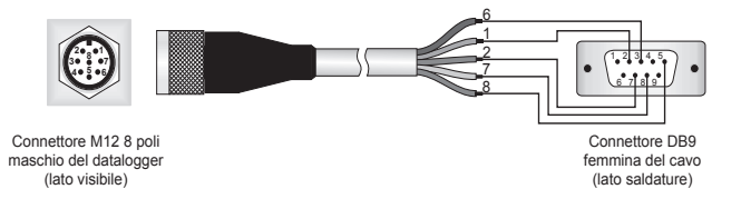
Fig. 3: Collegamento del cavo CP2013-DB al pluviometro
