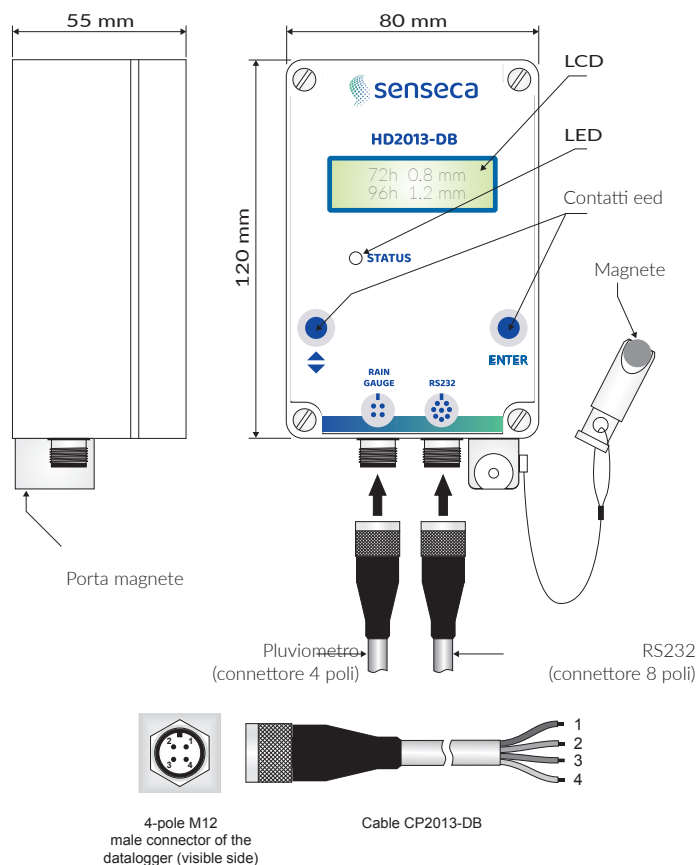
Fig. 2: Descrizione e connessioni
