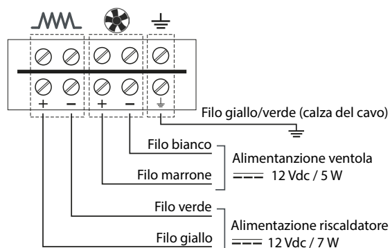
Fig. 1 - corrispondenze tra morsetti e fili del cavo
