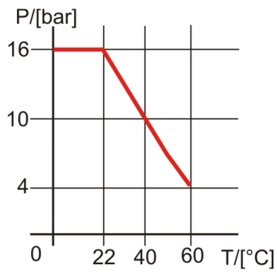
Diagrama de temperatura-presión PVC-U
