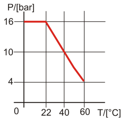
Temperatur-Druck-Diagramm PVC-U
